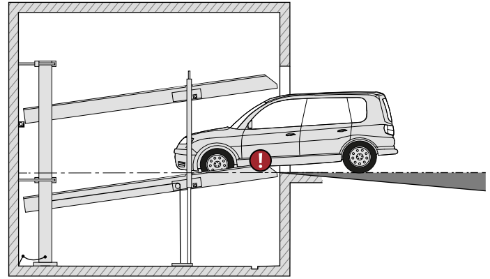
max. 2% gradient
